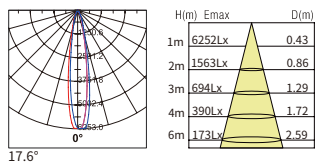
15° 33W
