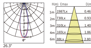
24° 15W
