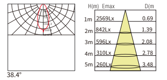
38° 30W
