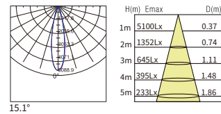
15° 12W
