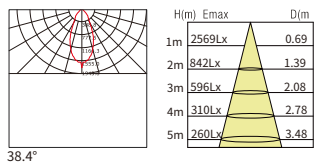
38° 30W
