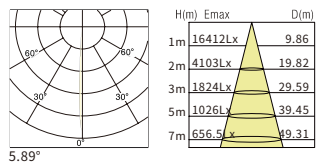
6° 10W
