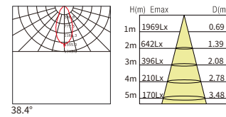
38° 20W
