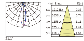
15° 25W
