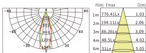
8W 36°
