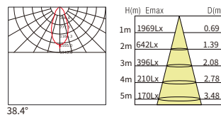
38° 20W
