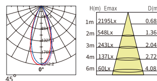
45° 15W
