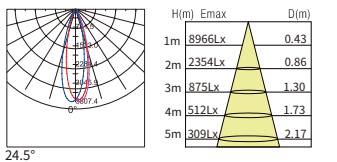
38° 25W
