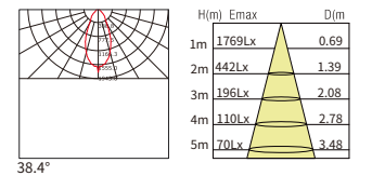
38° 12W
