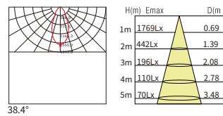
38° 12W
