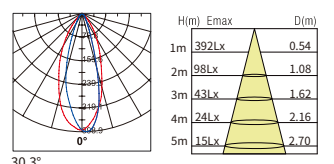
Elli. 30° 4W
