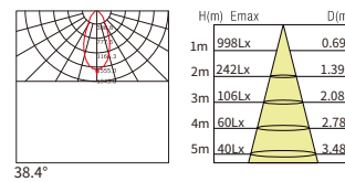
38° 7W
