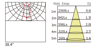
38° 30W
