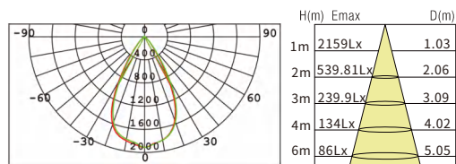
20W 60°
