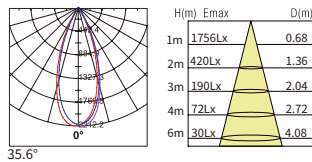
36° 15W
