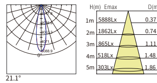
15° 15W
