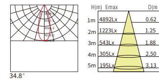
30° 28W
