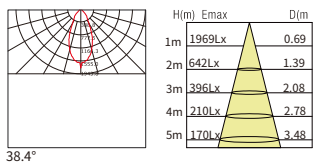
38° 20W
