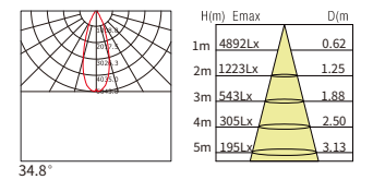
30° 28W
