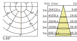
6° 10W
