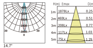
15° 8W
