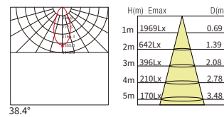
38° 20W
