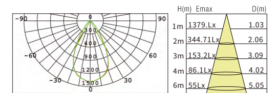
15W 60°
