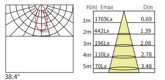
38° 12W
