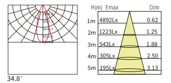
30° 28W
