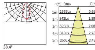
38° 30W
