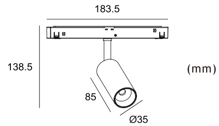
15° 8W
