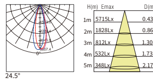
38° 15W
