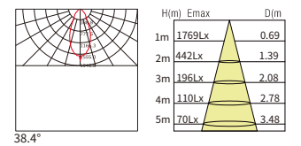
38° 12W
