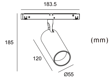
15° 15W
